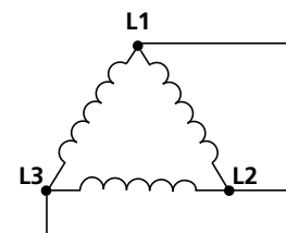
Delta ( \Delta )
